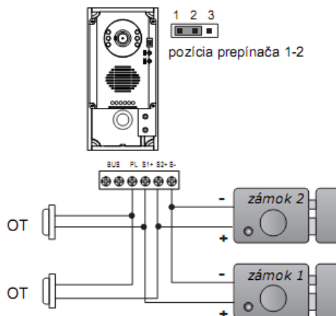
zapojenie dvoch zámkov
