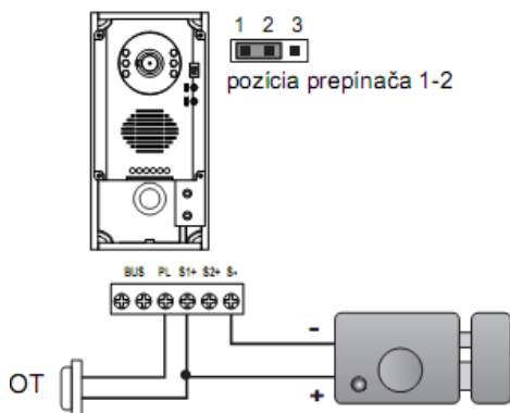
zapojenie jedného zámku
